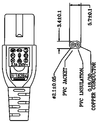
AC线剖面图
